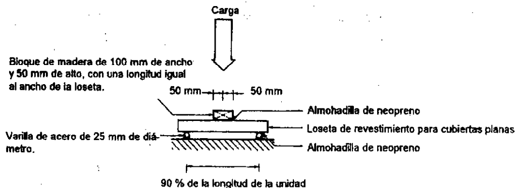
Figura 2. Disposición para el ensayo de resistencia a la flexión de losetas de revestimiento para cubiertas planas
