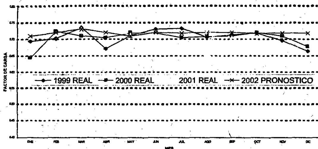
COMPARACIÓN DE PRONÓSTICO DE FACTOR DE CARGA PARA EDECHI S.A.
