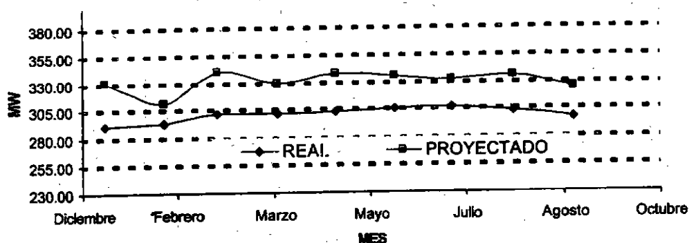
DEMANDA MAXIMA DE ELEKTRA REAL 2001 VS PROYECTADO
