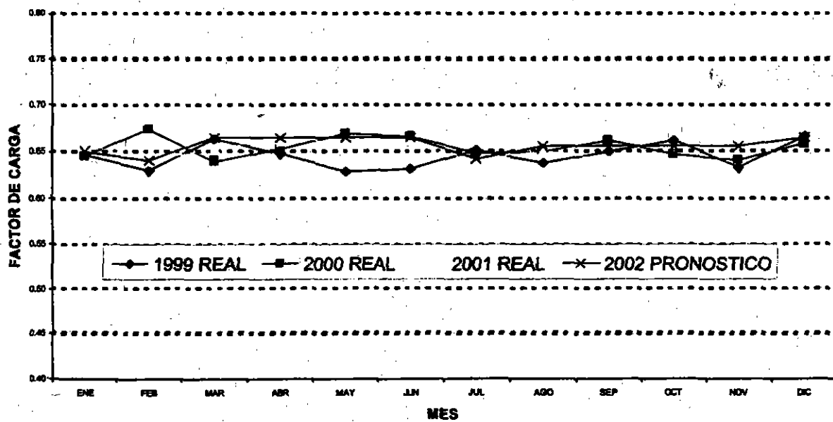
COMPARACIÓN DE PRONÓSTICO DE FACTOR DE CARGA PARA EDEMET S.A.
