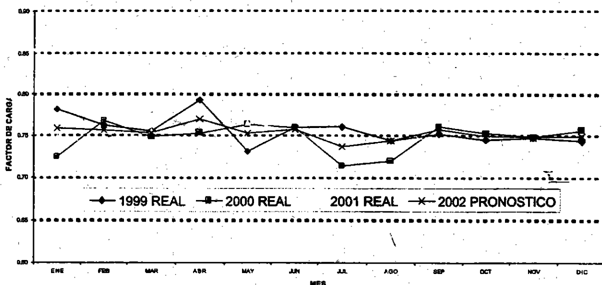
COMPARACIÓN DE PRONÓSTICO DE FACTOR DE CARGA PARA ELEKTRA S.A.
