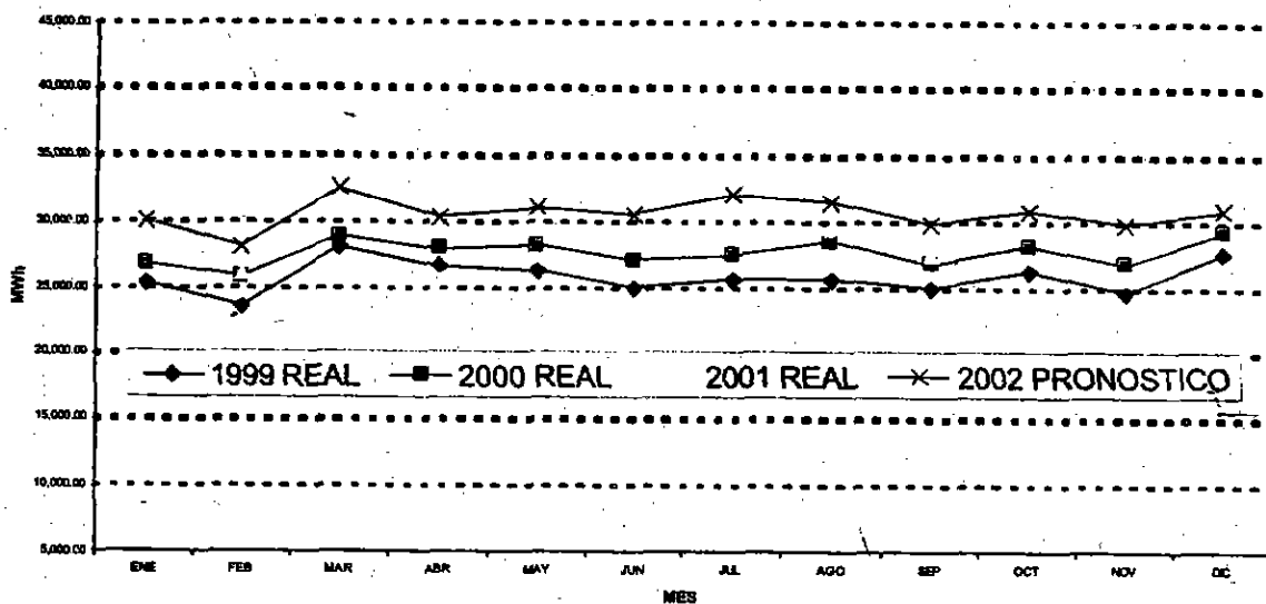
COMPARACIÓN DE PRONÓSTICO DE ENERGÍA PARA EDECHI S.A.
