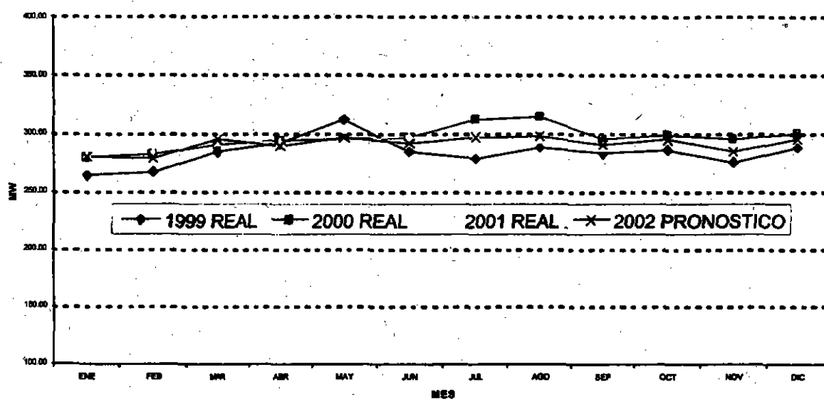
COMPARACIÓN DE PRONÓSTICO DE DEMANDA MÁXIMA PARA ELEKTRA S.A.
