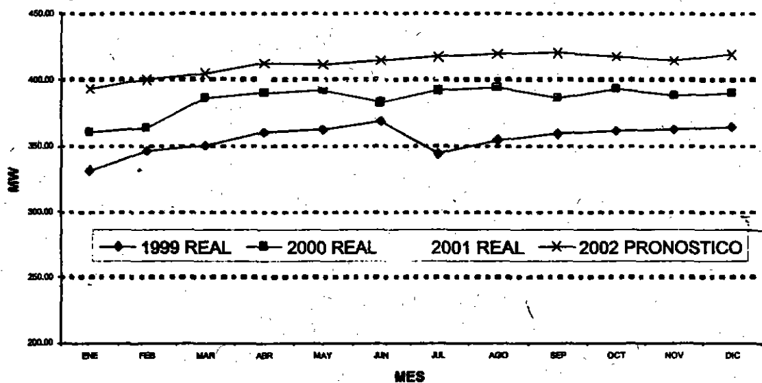
COMPARACIÓN DE PRONÓSTICO DE DEMANDA MÁXIMA PARA EDEMET S.A.
