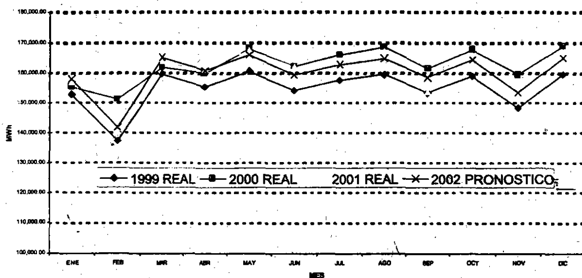
COMPARACIÓN DE PRONÓSTICO DE ENERGÍA PARA ELEKTRA S.A.
