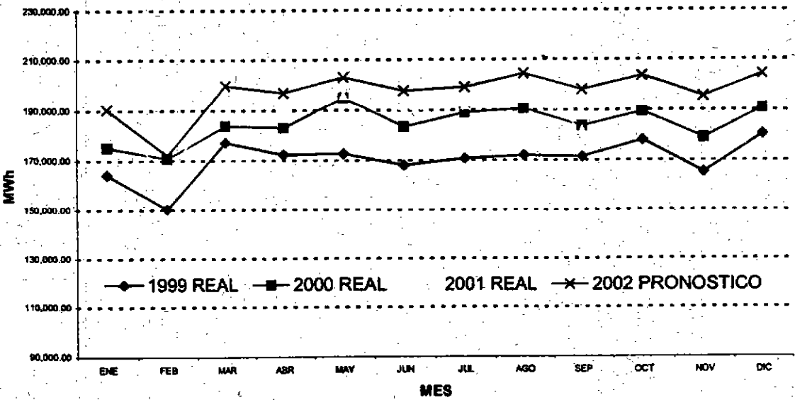
COMPARACIÓN DE PRONÓSTICO DE ENERGÍA PARA EDEMET S.A.
