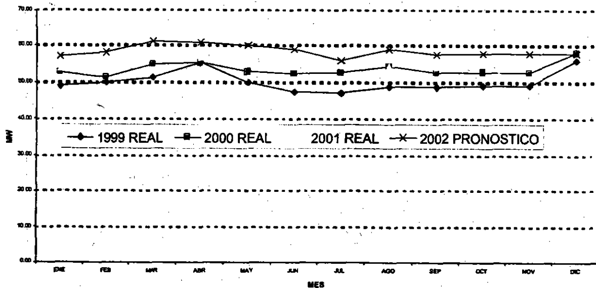
COMPARACIÓN DE PRONÓSTICO DE DEMANDA MÁXIMA PARA EDECHI S.A.
