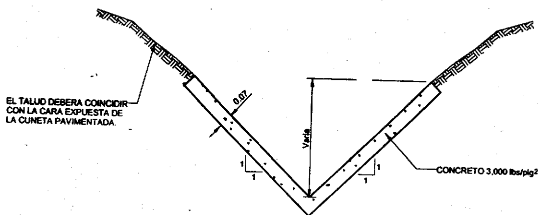
DETALLE DE CUNETA PAV. PROFUNDA EN "V"
