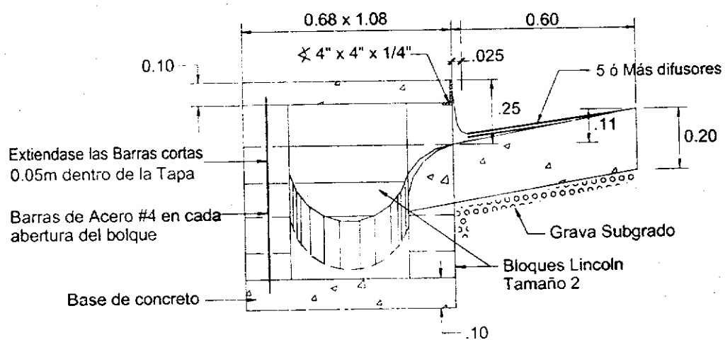
SECCION J
