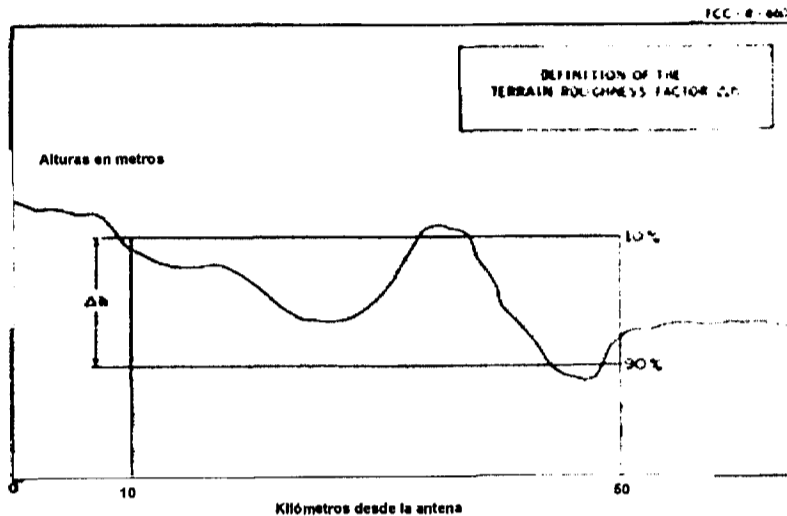
Figura 3.1. Definición del índice de rugosidad del terreno
