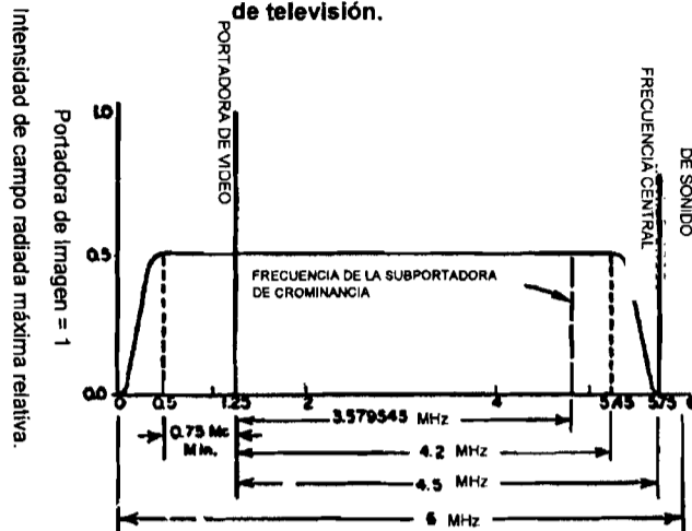
Figura 4.1. Característica de la emisión de la señal compuesta de televisión.
